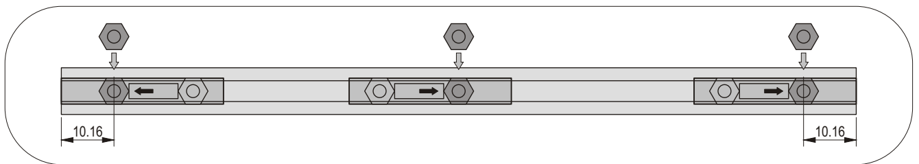
Gesamtfrentplatte
