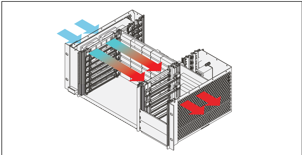
Figure 5: Entwärmung
