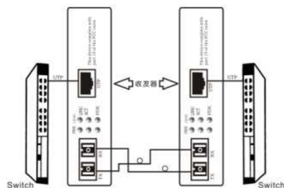
Figure 6.1 Schéma de connexion MC
