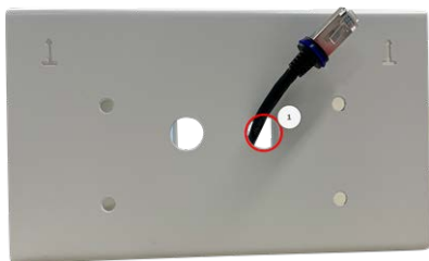
Abb. 11: Netzwerkverkabelung vorbereiten
