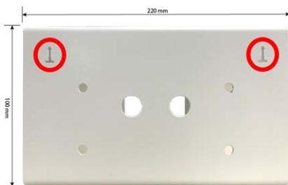
Abb. 9: Abmessungen Q71Corner/Pole Mount – Vorderansicht
