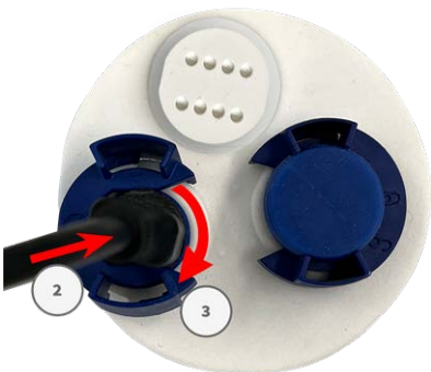
Abb. 15: Drücken Sie den Stecker fest ein, bis der blaue Dichtring einrastet.
