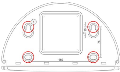
Abb. 7: Wall Mount mit Bohrungen zur Positionierung der Befestigungsschrauben
