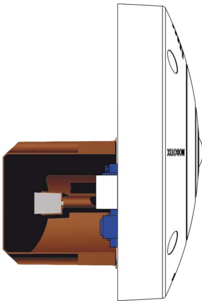
Abb. 5: Seitenansicht der Q71 über Unterputzsteckdose
