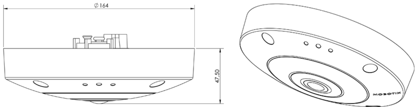
Abb. 4: Q71: Alle Maßangaben in mm
